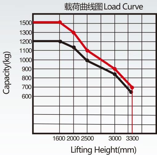
TW12JB-070E TW15JB-070E
